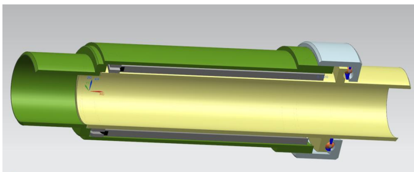
КОМПЕНСАТОР КРУТИЛЬНЫХ ПЕРЕМЕЩЕНИЙ
